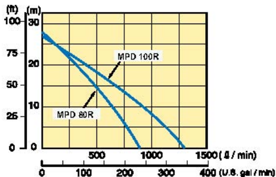
Curba de debit si presiune:
